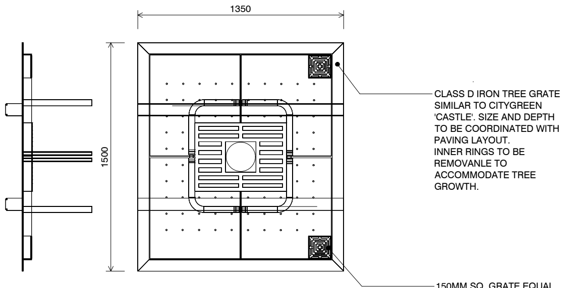
ELEVATION - SIDE 1:25
