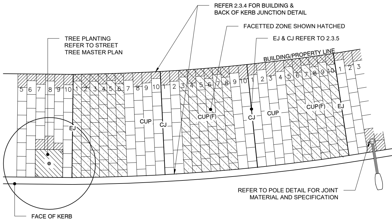
PLAN 1:100
