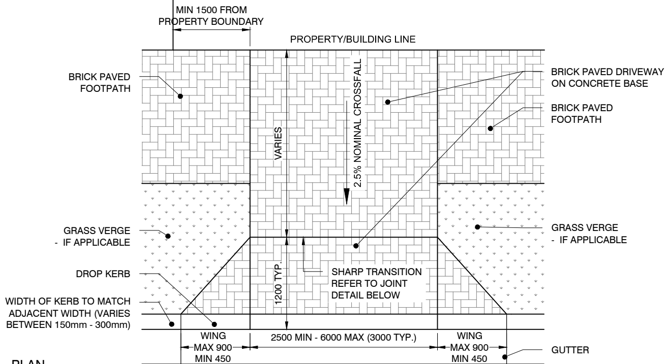
PLAN 1:50
