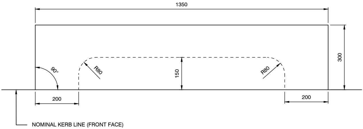
PLAN 1:10
