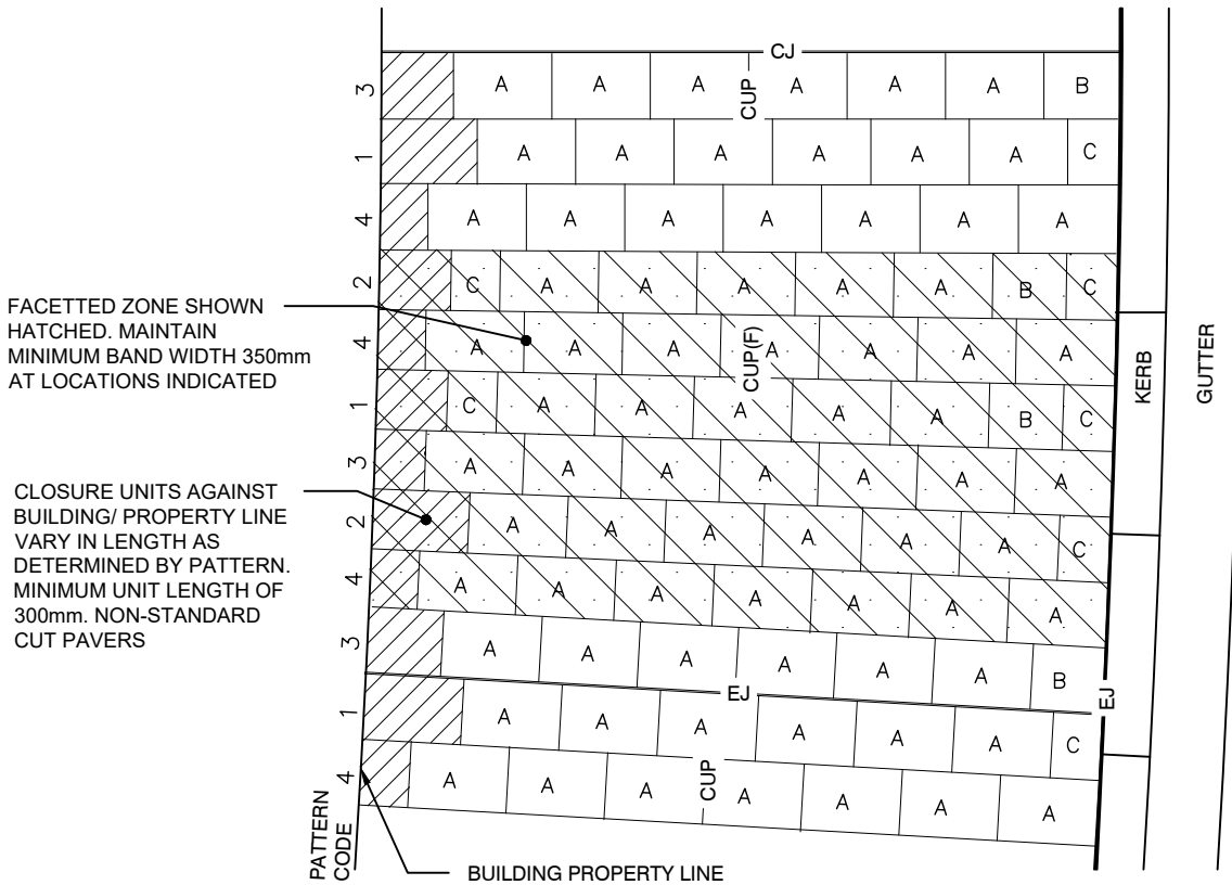
PLAN 1:100
