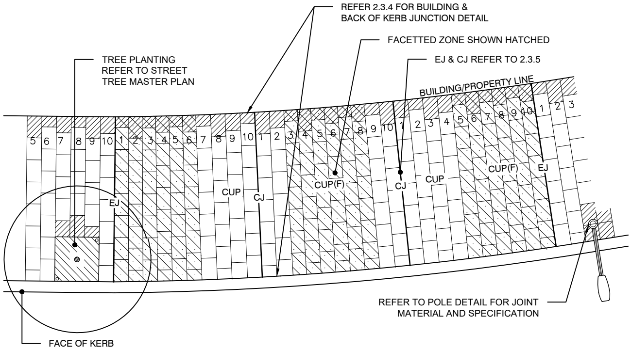
PLAN 1:100
