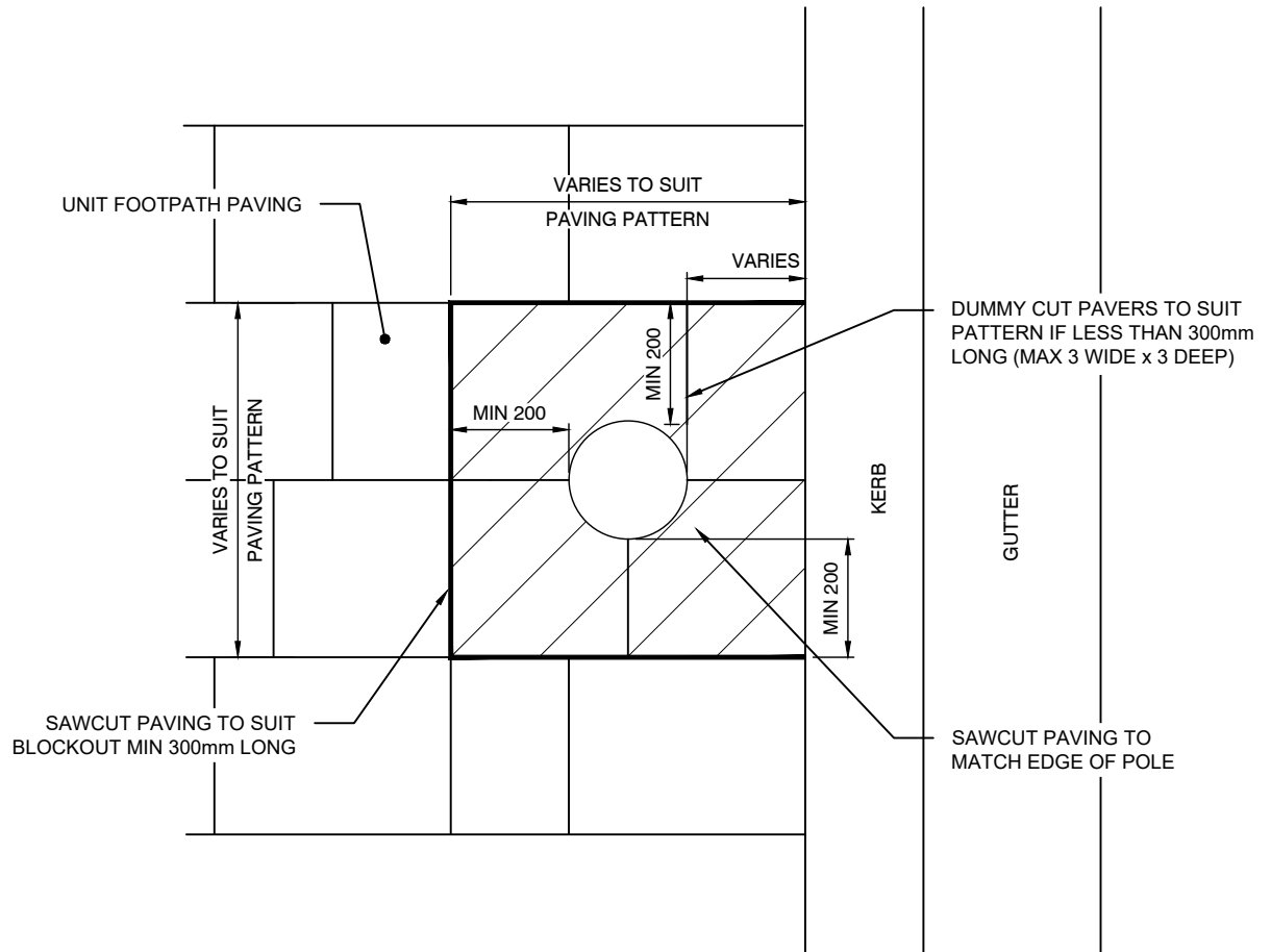
PLAN 1:20
