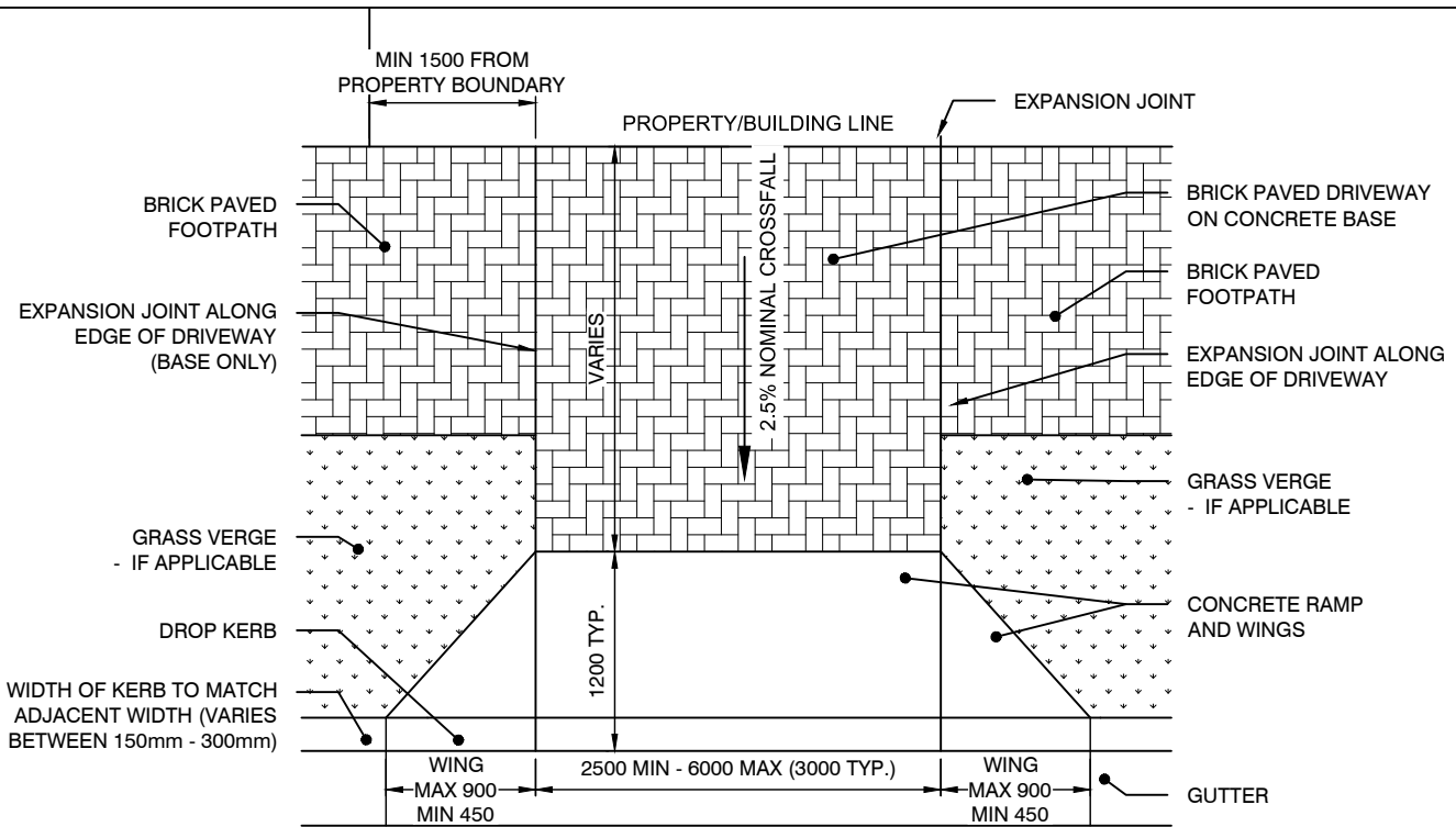
PLAN 1:50
