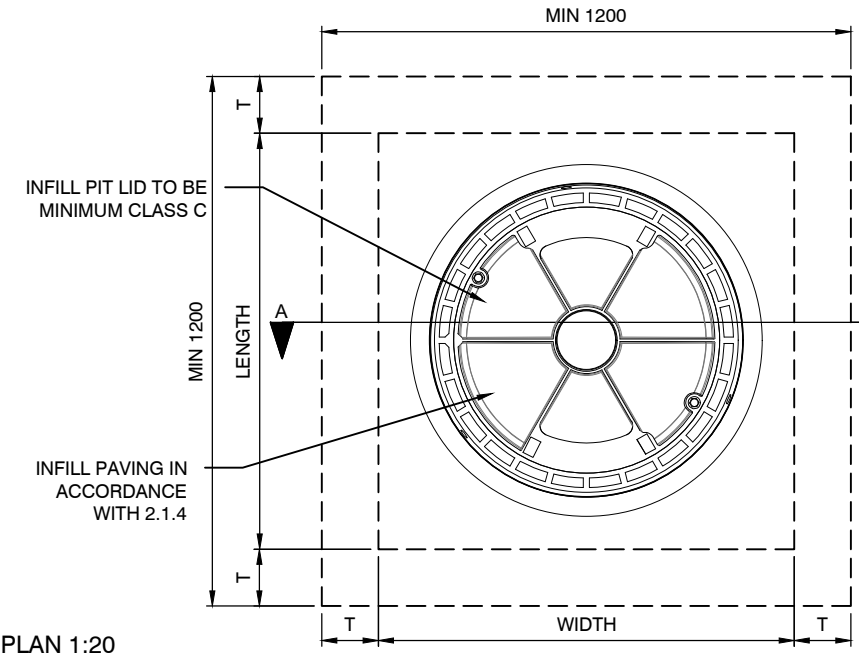
PLAN 1:20
