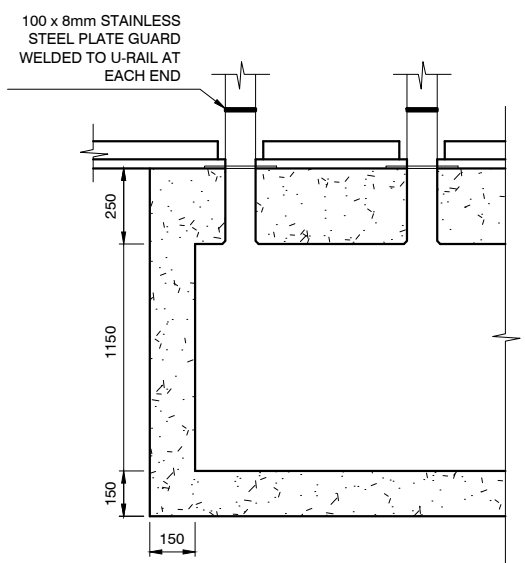
SECTION A-A 1:25
