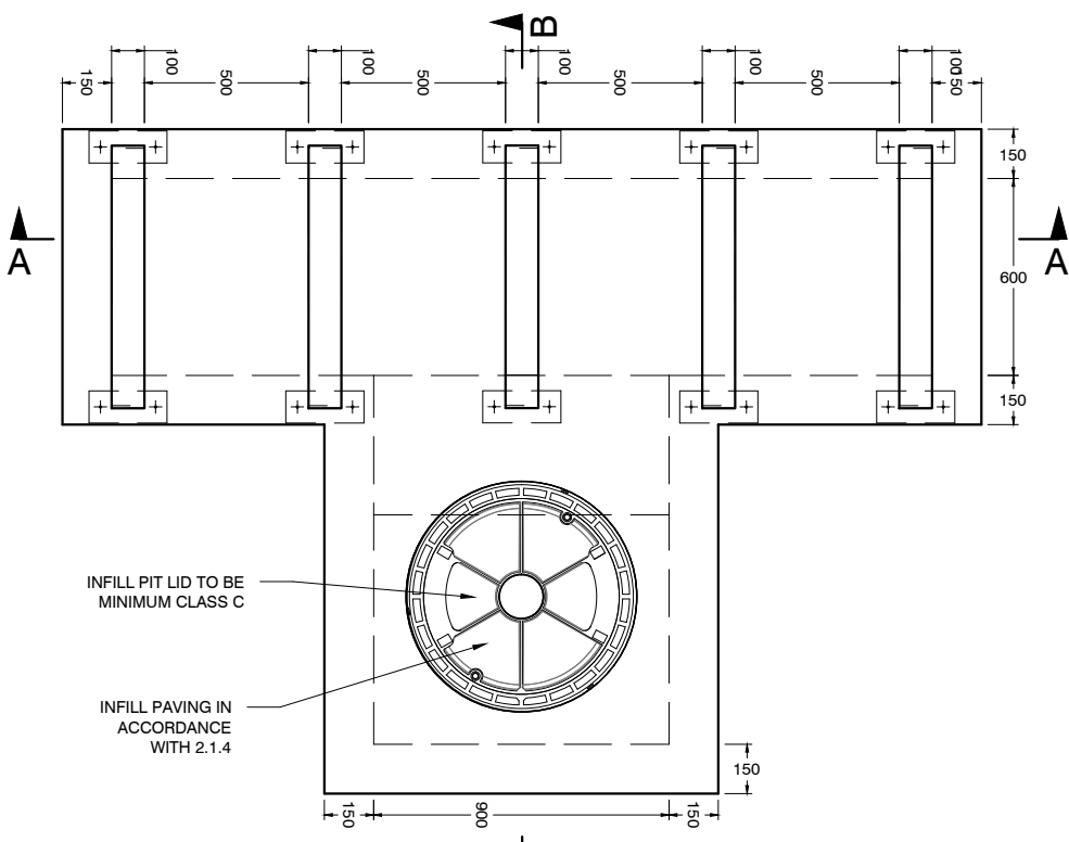
PLAN 1:25
