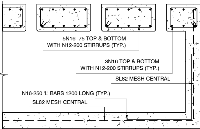
SECTION A-A 1:25
