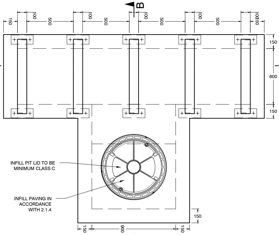
PLAN 1:25
