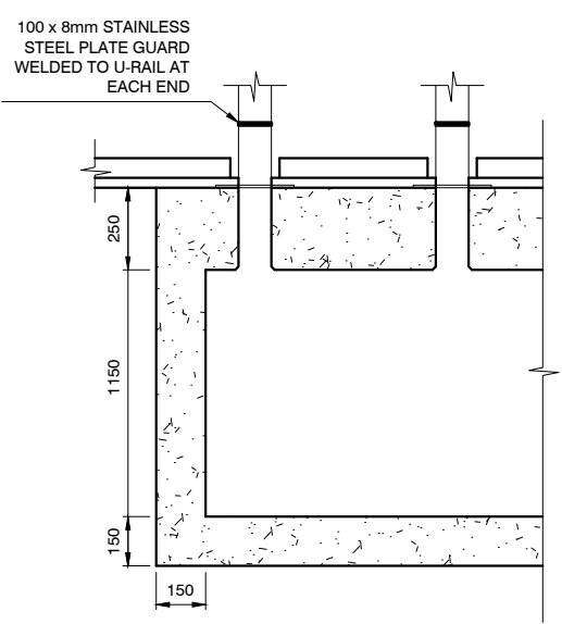
SECTION A-A 1:25
