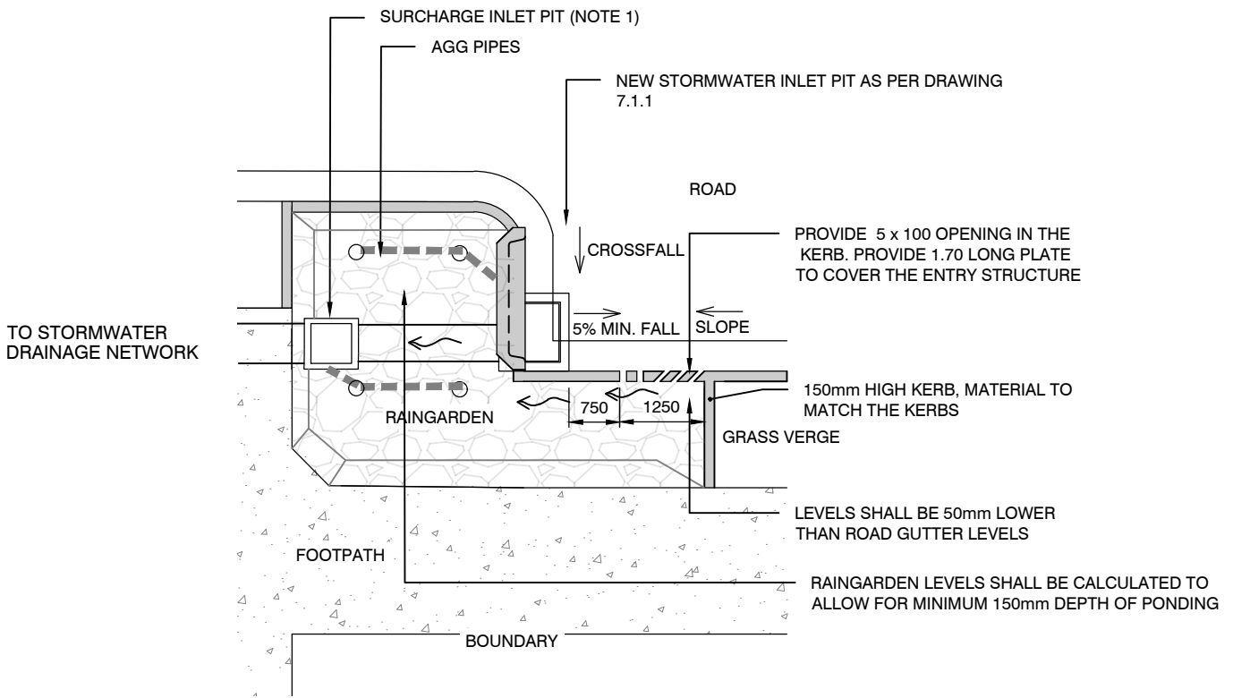
PLAN 1:100
